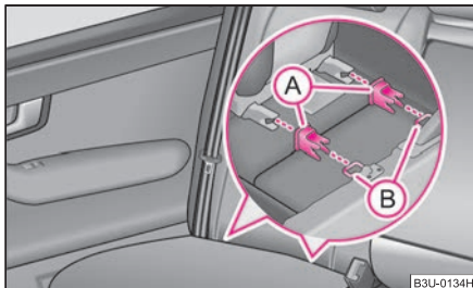
Obr. 128 Upevňovací oka (systém ISOFIX)
