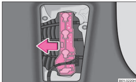
Obr. 181 Demontáž tělesa držáku žárovek (Combi, Sedan)
