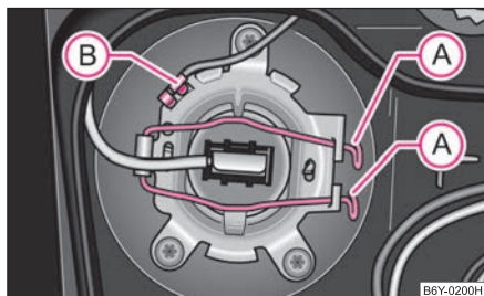
Obr. 172 Demontáž žárovky dálkového světla
